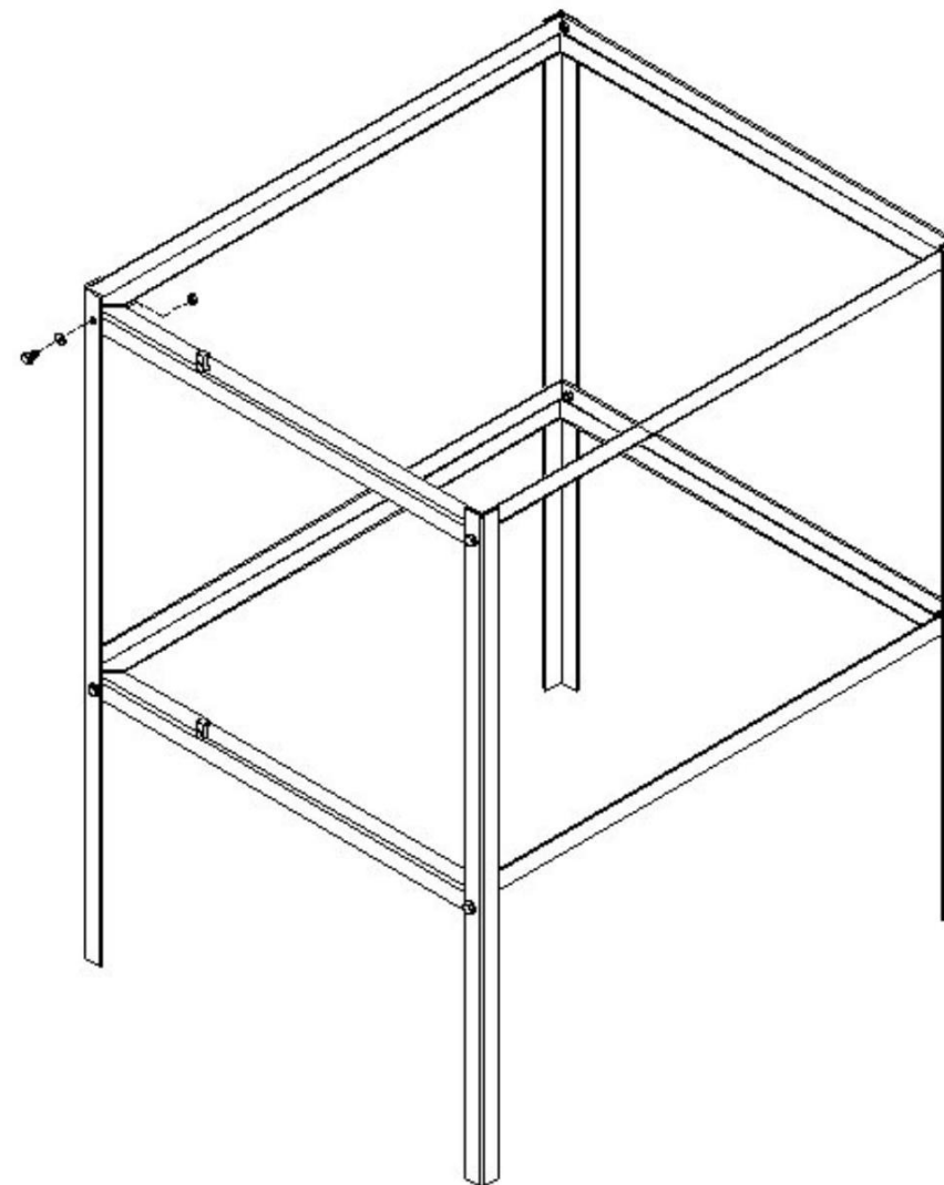
VISTA DE MONTAGEM (ESTRUTURA DO MARMITEIRO INDUSTRIAL)
